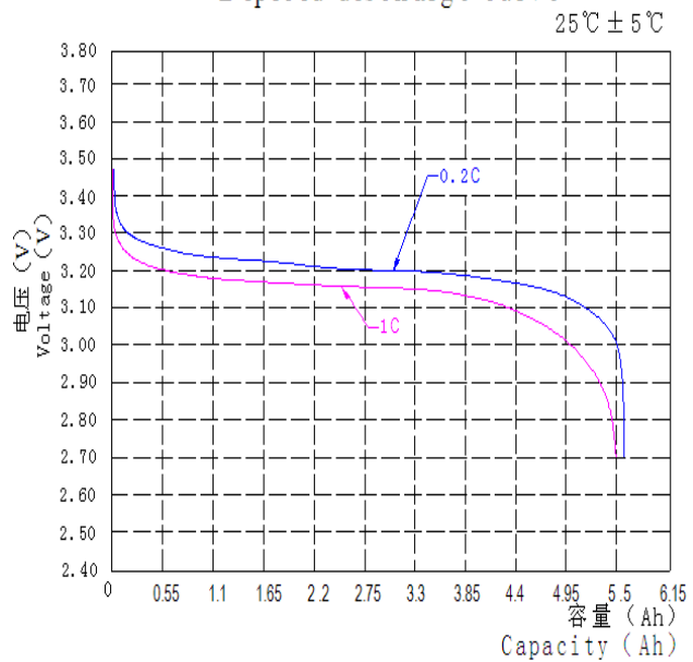
放电曲线图 Diploid discharge curve
