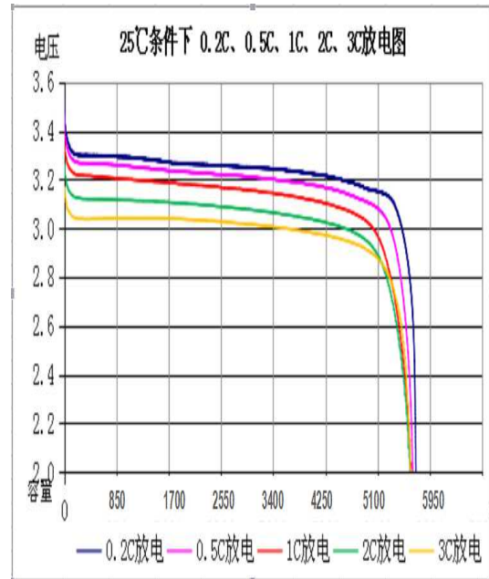
放电曲线图 Diploid discharge curve
